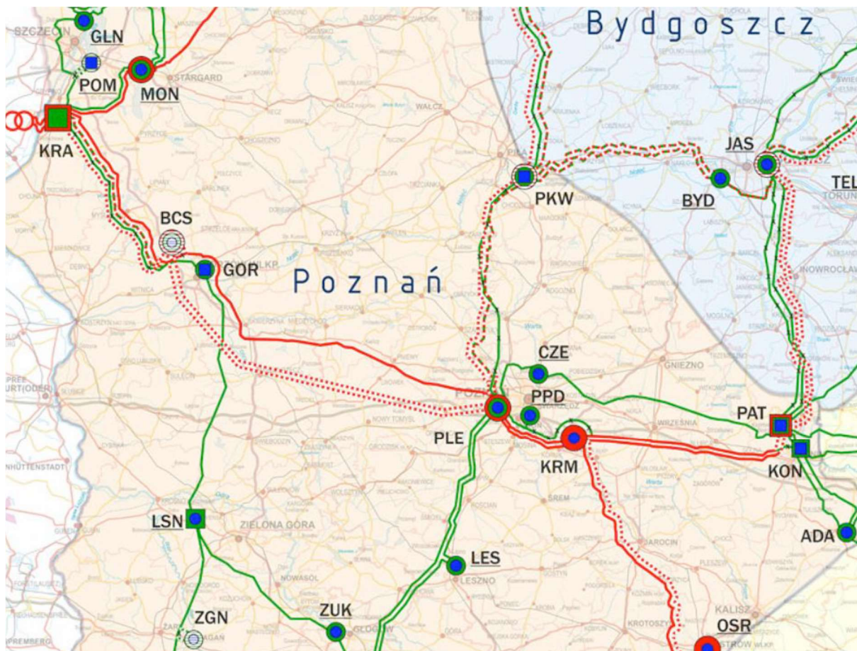
Rycina 13. Sieć przesyłowa energii elektrycznej na terenie województwa wielkopolskiego
